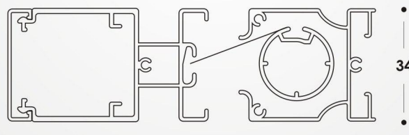
sistema completo sistema completo complete system système complet
